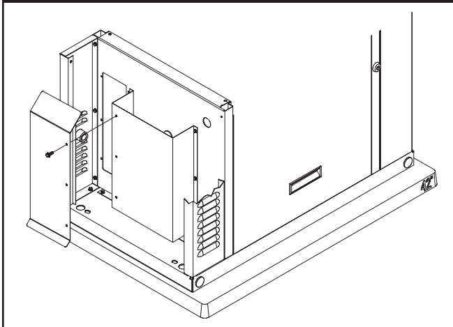
Figura 27 — Acceso a la Parte Trasera del Panel de Control
